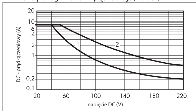
H 50 - Obciążenie graniczne dla prądu stałego (dla DC1)
