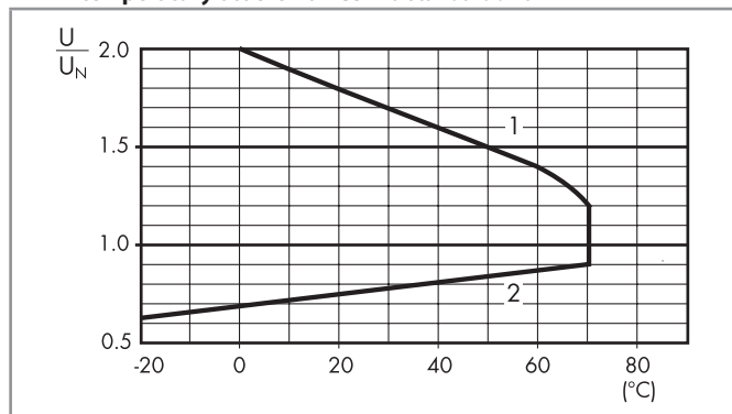
R 50 - Dopuszczalny zakres napięcia pracy cewki w zależności od temperatury otoczenia - Cewka standardowa
